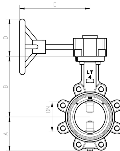
Type AF
